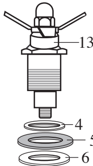
013304 NSF Sseal
