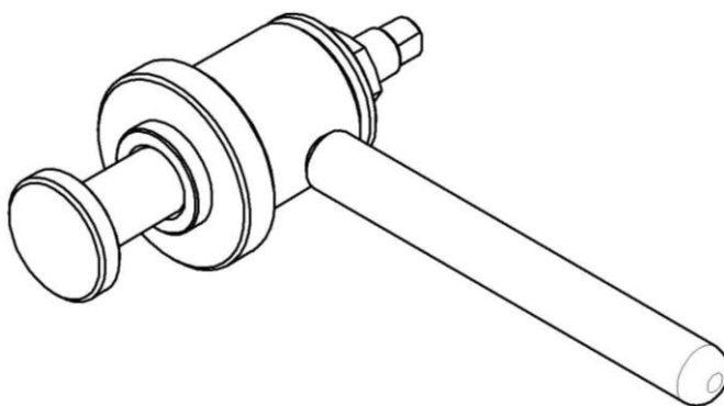
Рис. 8. Приспособление для запрессовки манжет.
