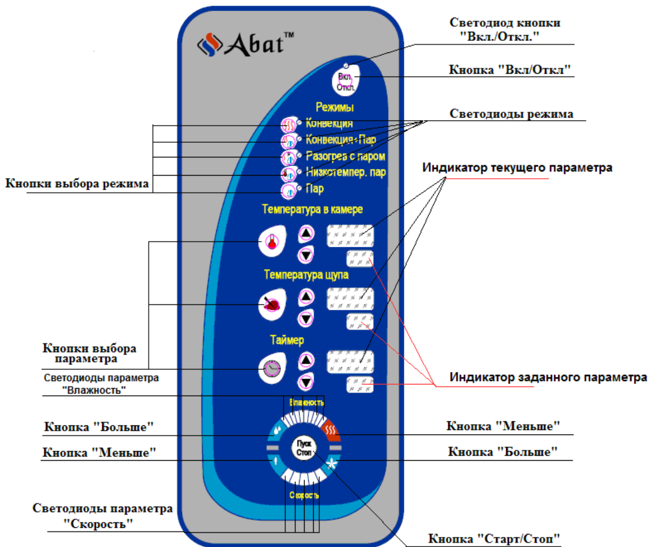
Рис. 3. Пленочная клавиатура
