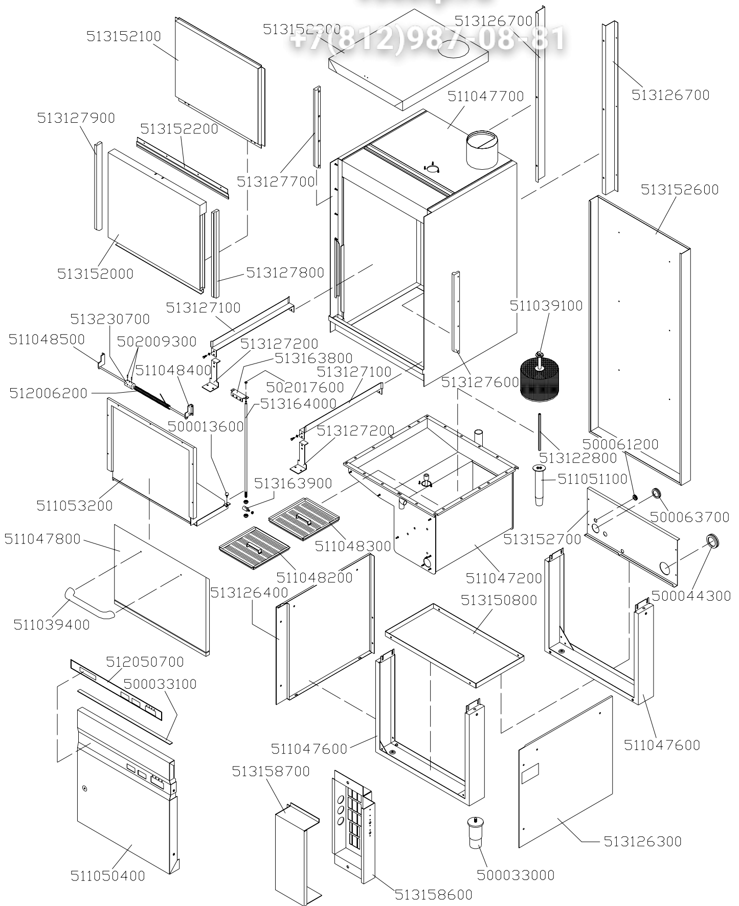
MLP60E_esterno
