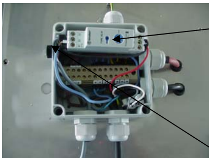
Multifunktionsrelais / multifunctional relais Teile-Nr. 3104131 (S2 Anschlusskabel länger abisolieren / more insulation of cable S2 has to be removed) rückfallverzögert Werkseinstellung 60 Sek. release delay, set, set ex factory 60 sec.
