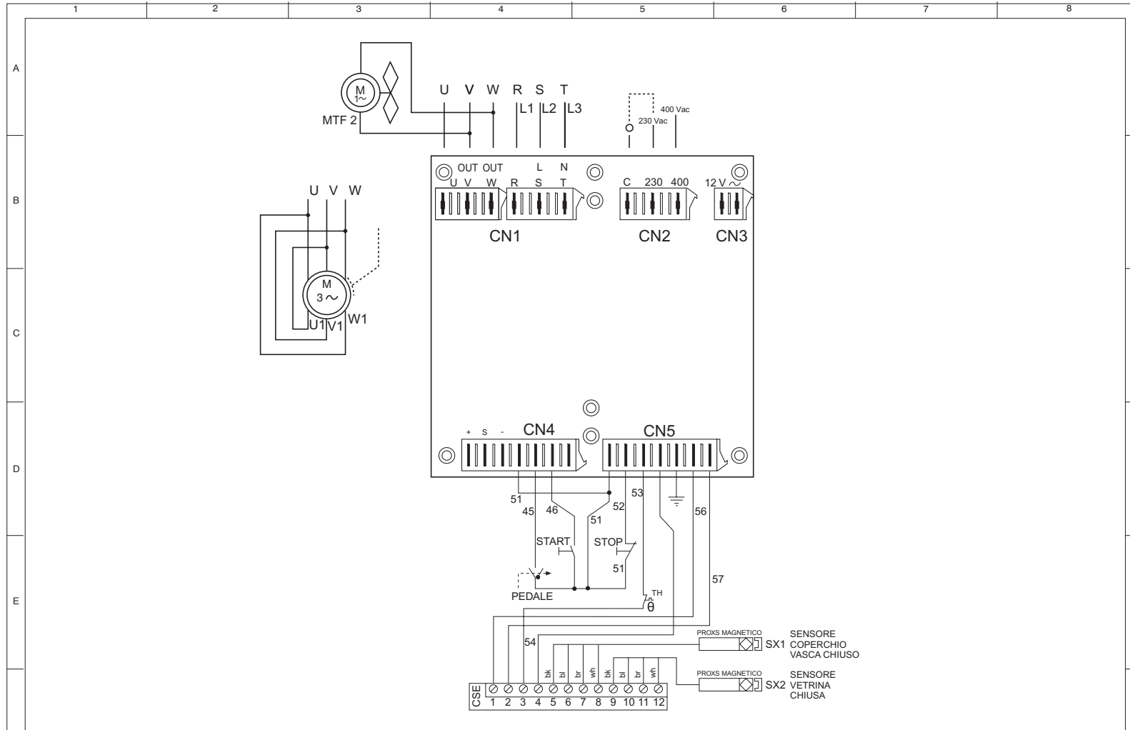
Schema elettrico trifase (230/3) / Three-phase wiring diagram / Schéma électrique trifasée Dreiphasenschaltplan / Esquema eléctrico trifásica C/E652-653
